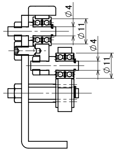
断面図 A-A
